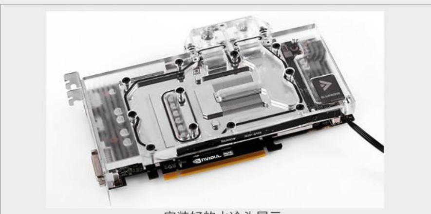
安装好的水冷头展示
