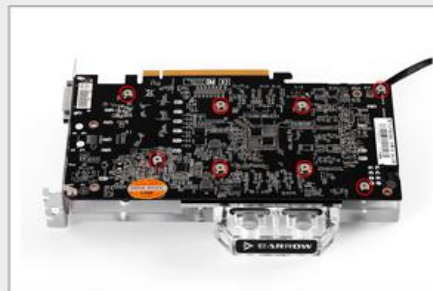
4.安装图中标红位置螺丝
